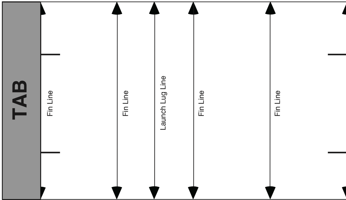
T-60 Four Fin Tube Marking Guide
